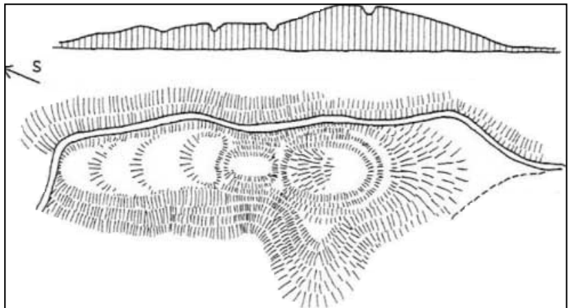
Plán hradu nad Velkým Březnem podle Josefa Nittnera, pořízený před rokem 1931. Plán lokality dole, nahoře podélný řez.
